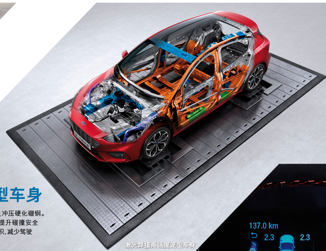
激光焊接高强度笼型车身
